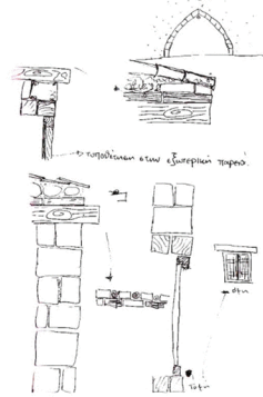
Εύλινες κατασκευές
